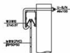
상세도 "A"
