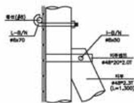
상세도 "B"
