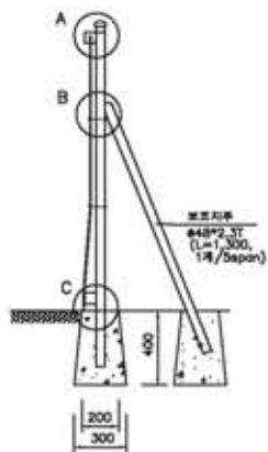
펜스 측면도
