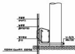
상세도 "C"
