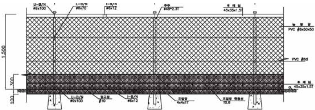
야생동물유도펜스 (H1.5) 정면도
